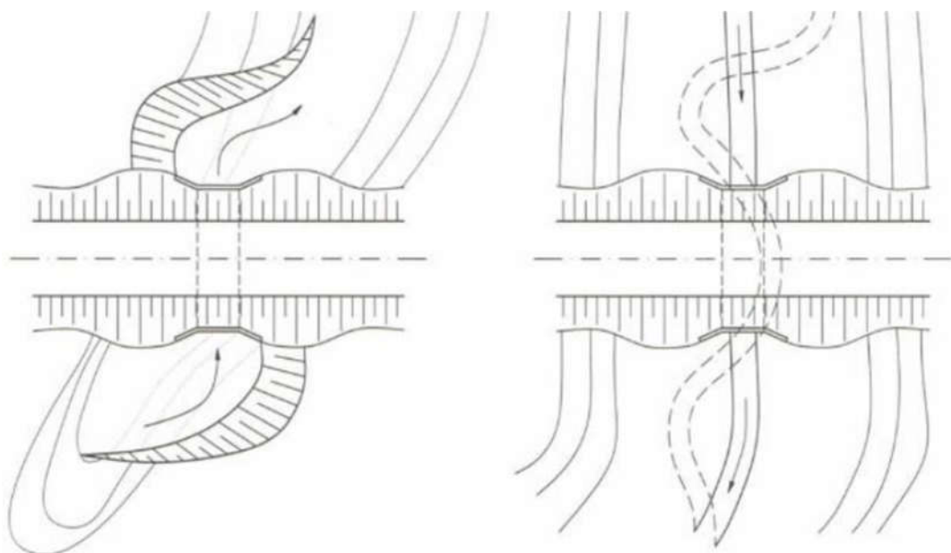
Slika 5. Regulacija vodotoka na dva načina[3]
