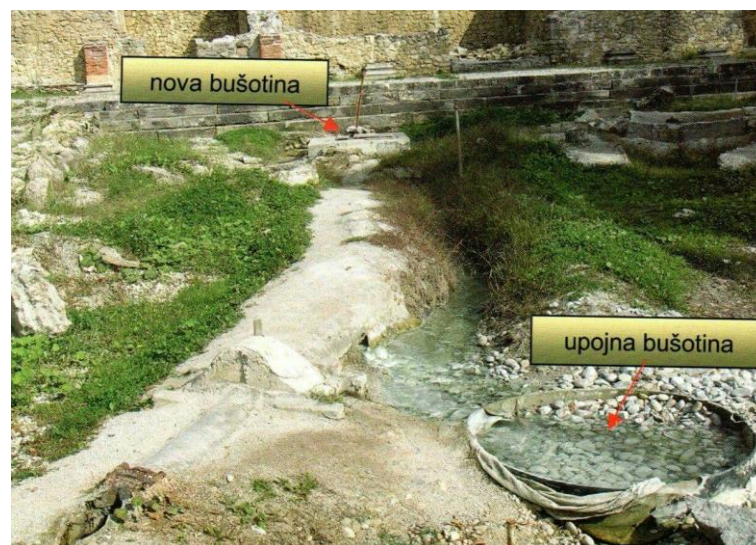
Slika 3.5. Detalj izvorišta s novom kaptadžom i „upojnom bušotinom“
