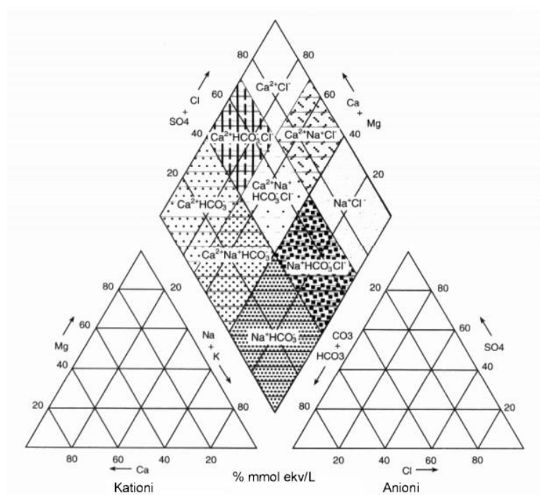
Slika 2.2. Prikaz vodnih facijesa u rombu Piperova dijagrama
