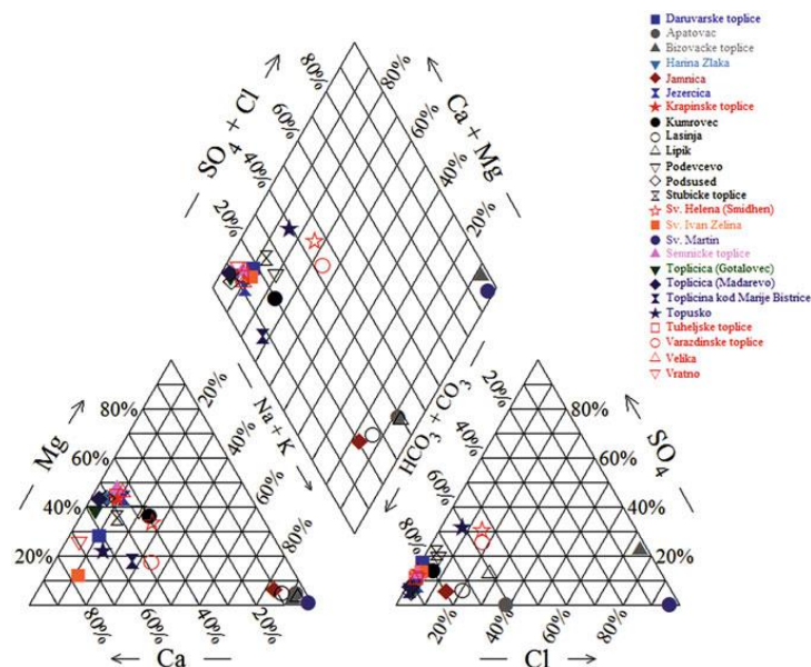
Slika 3.4. Piperov dijagram osnovnog ionskog sastava Varaždinskih toplica u usporedbi s ostalim termomineralnim vodama sjeverozapadne i istočne Hrvatske
