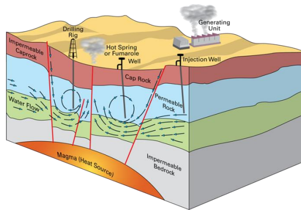
Slika 2.1. Pojednostavljen prikaz geotermalnog sustava
