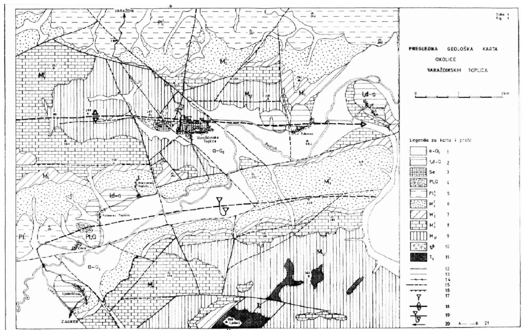
Slika 3.2. Pregledna geološka karta okolice Varaždinskih toplica
