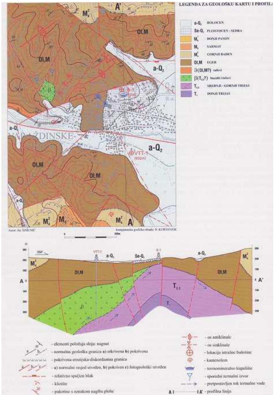
Slika 3.3. Geološka karta i geološki profil okolice Varaždinskih toplica
