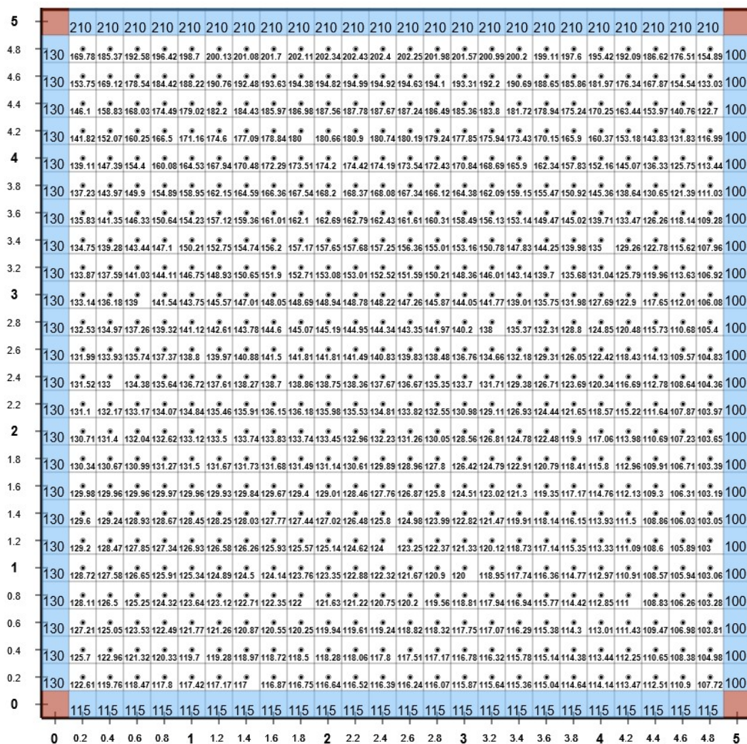
Slika 3. Problem dužine 5, širine 5 s razmakom između čvorova 0,2
