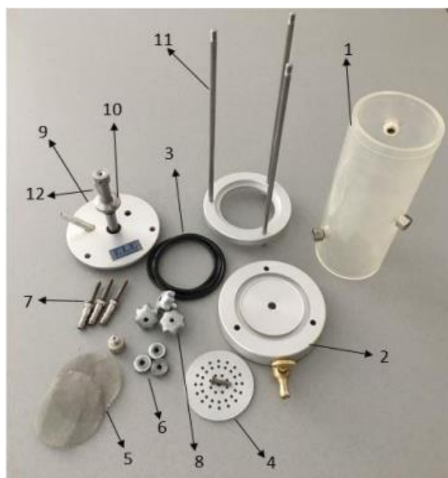
Slika 12. Dijelovi permeamtra [17]
