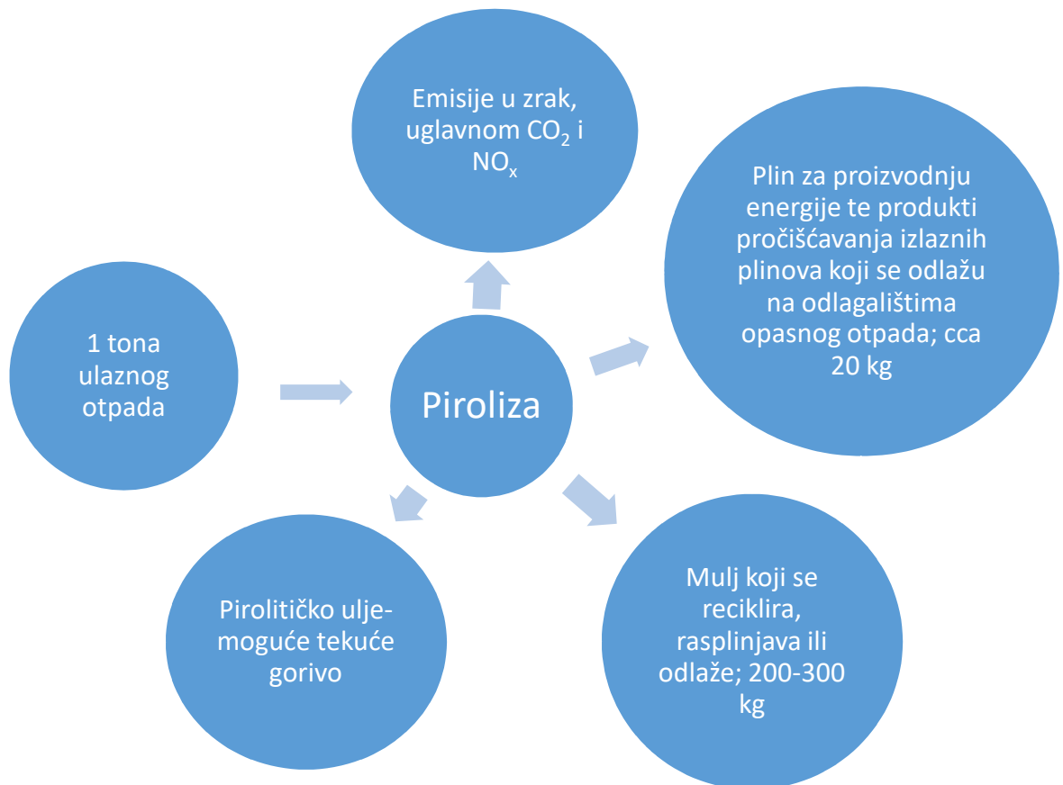
Slika 2 Produkti pirolize [8]
