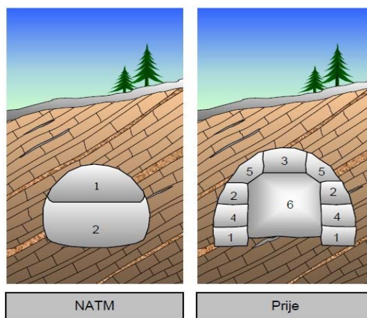
Slika 3.17 Pravovremeno zatvaranje podgradnog prstena[14]
