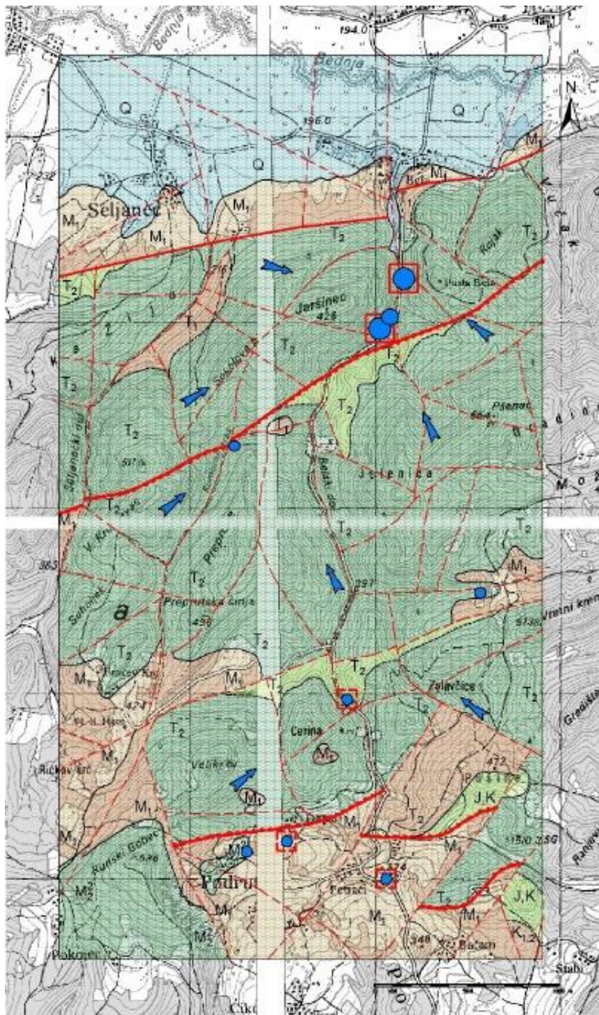
Slika 7. Hidrogeološka karta područja Belski dol (RGN 2008)
