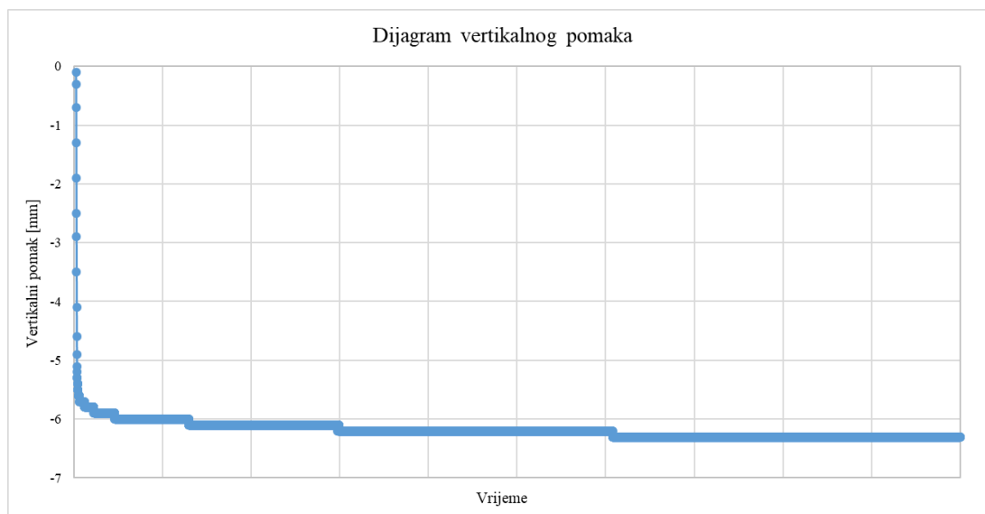
Slika 18. Dijagram vertikalnog pomaka
