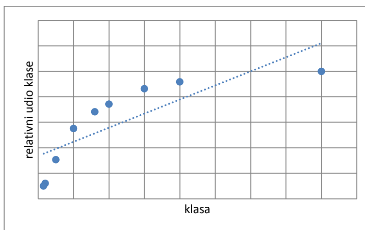
Slika 4: Grafički prikaz linearnog pravca regresije
