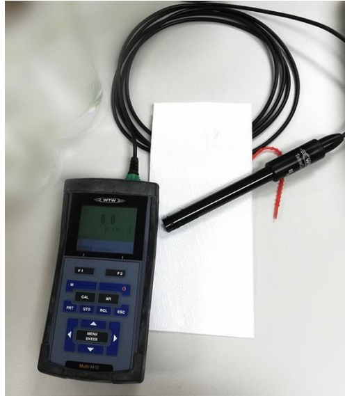
Slika 12 Više-parametarski mjerni instrument MultiLine® Multi 3410 IDS
