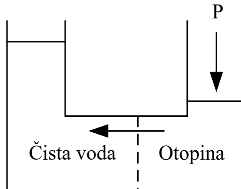
Slika 23. Reverzna osmoza [4]
