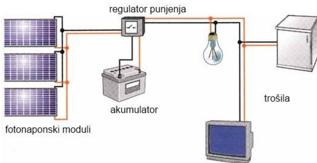
Slika 4. Prikaz samostalnog solarnog fotonaponskog sustava
