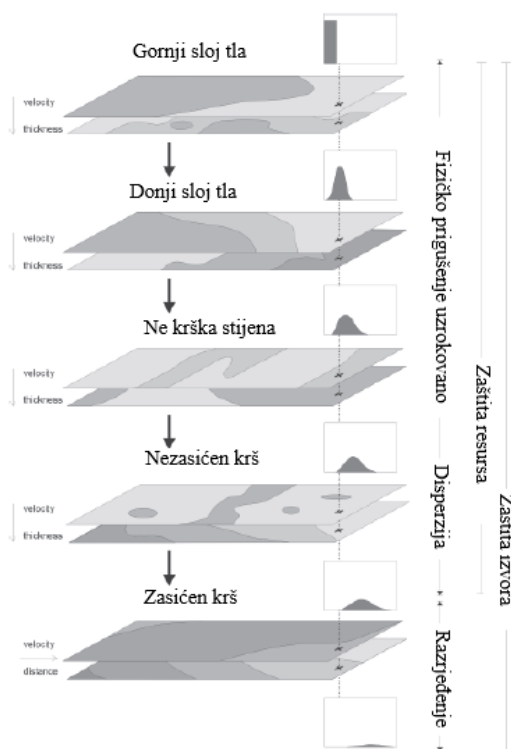
Slika 12. Metodologija preslikavanja vremena prijenosa VULK metodom (Zwahlen, 2004)
