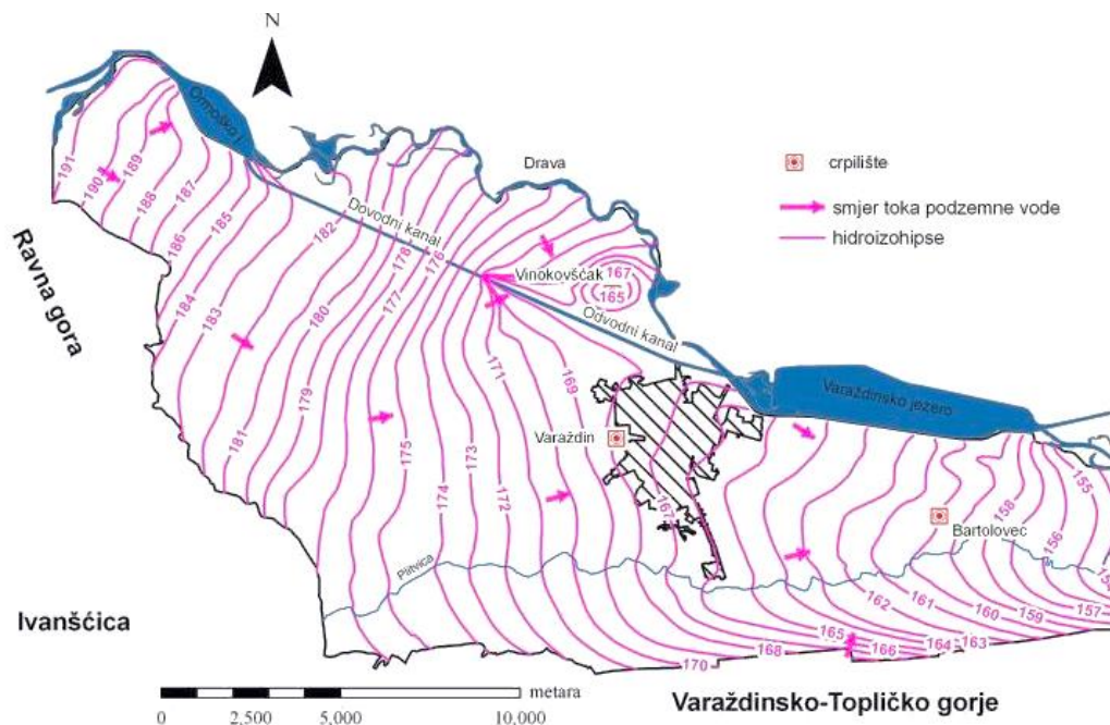
Slika 1. Varaždinski vodonosnik s crpilištima Varaždin, Bartolovec i Vinokovščak (Brkić i sur. 2012)
