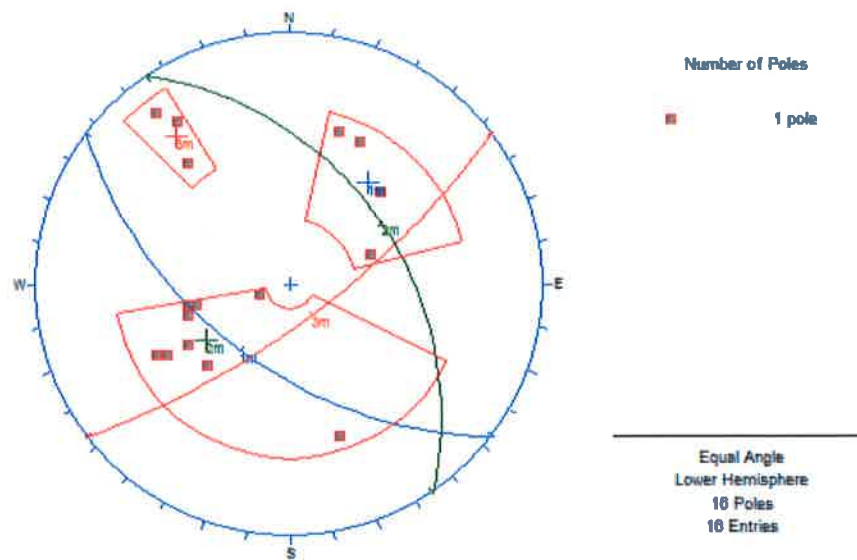
Slika 16. Kumulativni dijagram trasa ravnina pukotina i rasjeda mjerjen u zoni Kule Minčeta jedinice, slojni diskontinuiteti - zeleno, osna ravnina – plavo, okomito na os „b“ - crveno.
