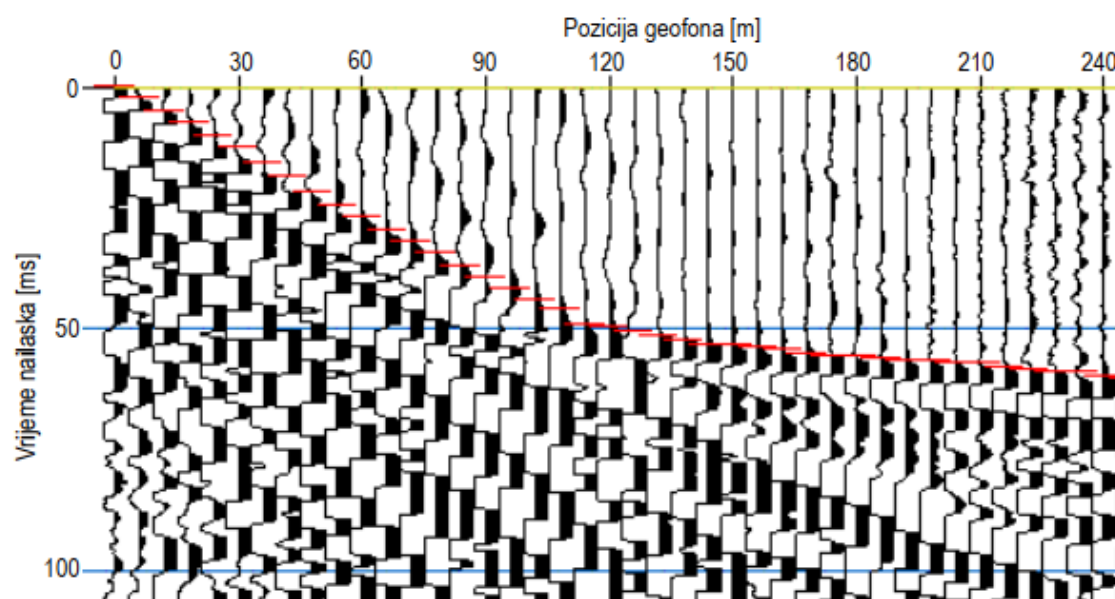
Slika 17 Vremena prvih nailazaka seizmičkih valova na geofone (crveno označeno). [6]
