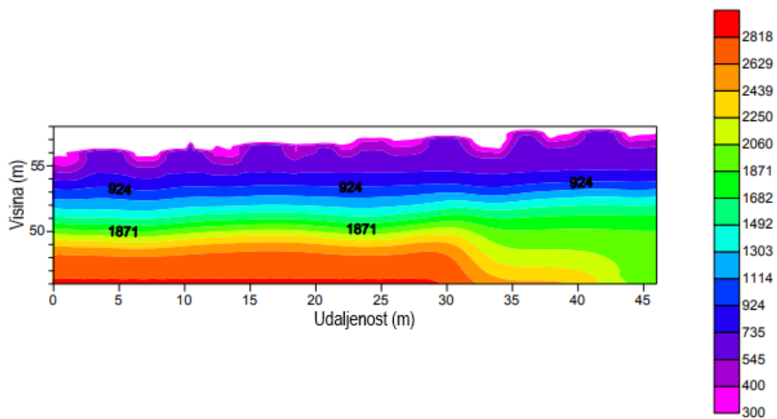
Slika 22 Model brzina za drugi profil (L2). [2]
