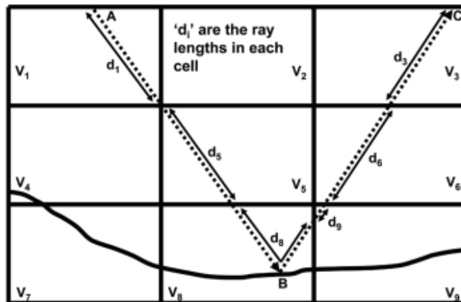
Slika 13 Podjela modela na ćelije u kojima svaka ćelija ima svoju vlastitu brzinu širenja vala. [3]
