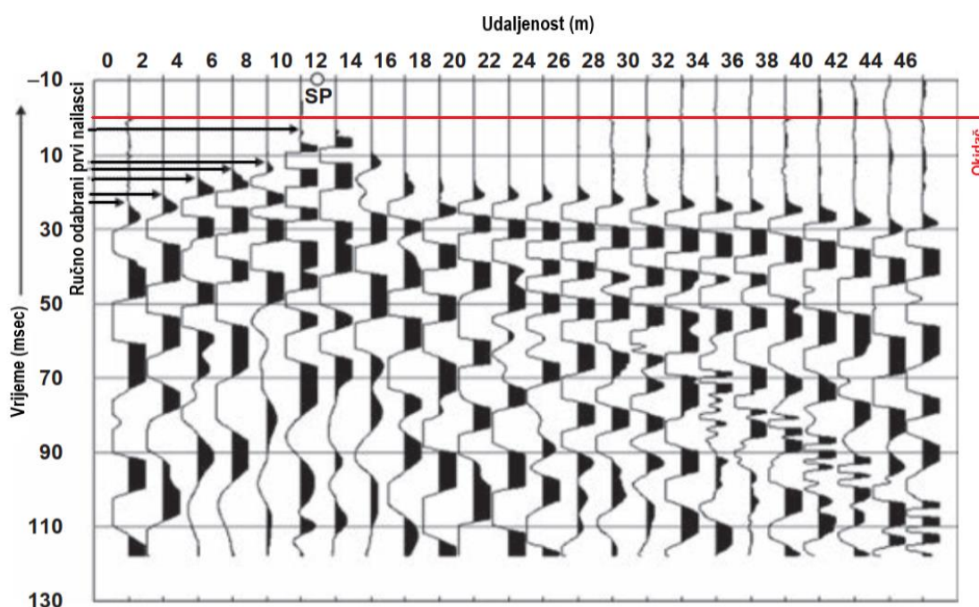
Slika 10 Seizmički tragovi u metodi refrakcije. [1]
