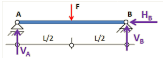
Slika 20. Zamjena oslonca s reakcijama
