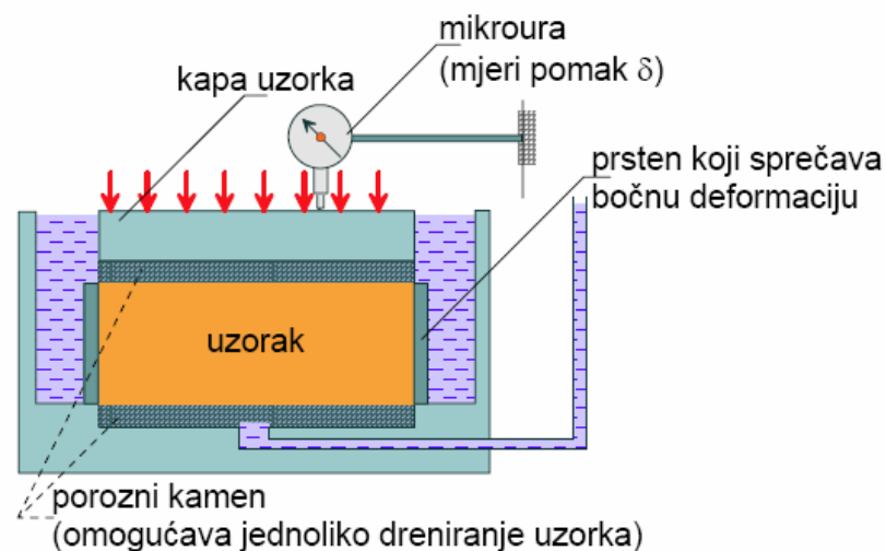
Slika 7. Shema edometra [6]
