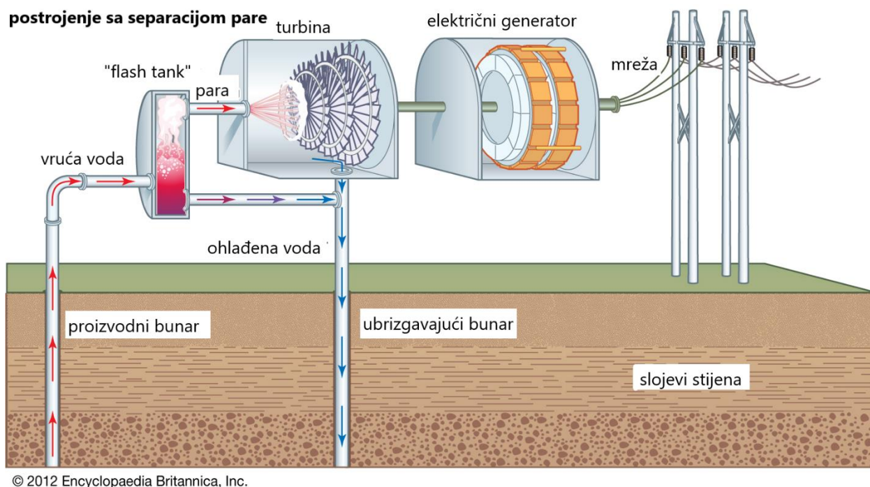
Slika5. Postrojenje sa separacijom pare [18]
