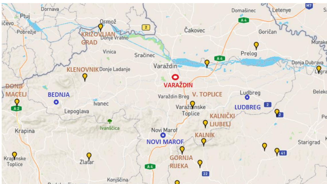
Slika 3. Kišomjerne (narančasta boja), klimatološke (plava boja) i glavna meteorološka postaja (crvena boja) u slivu rijeke Bednje i Plitvice (izvor: https://meteo.hr/ )
