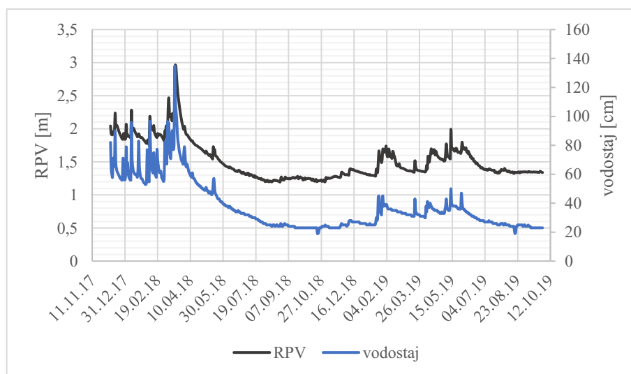
Slika 17. Grafički prikaz odnosa razine podzemne vode na vodocrpilištu Boljkovac i vodostaja na hidrološkoj postaji Boljkovac na vodotoku Miljašić Jaruga
