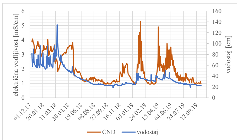
Slika 22. Grafički prikaz odnosa električne vodljivosti na vodocrpilištu Boljkovac i vodostaja na hidrološkoj postaji Boljkovac na vodotoku Miljašić Jaruga
