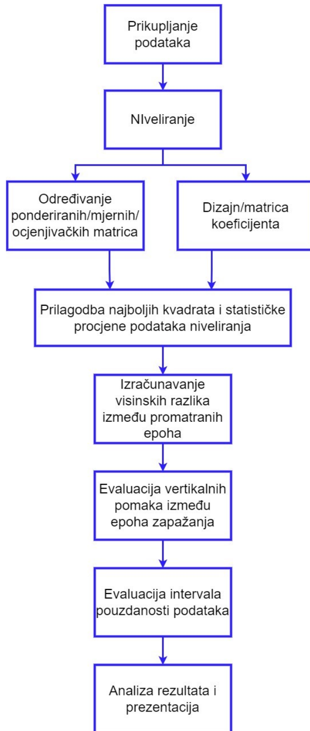
Slika 11. Metodologija niveliranja [31]
