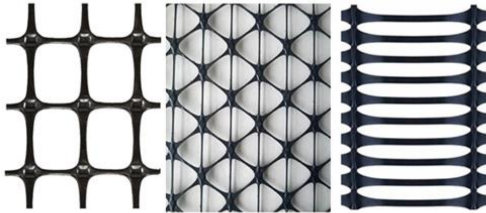
Slika 5. Različite vrste geomreža (a) dvoosna geomreža, (b) troosna geomreža, (c) jednoosna geomreža [10]
