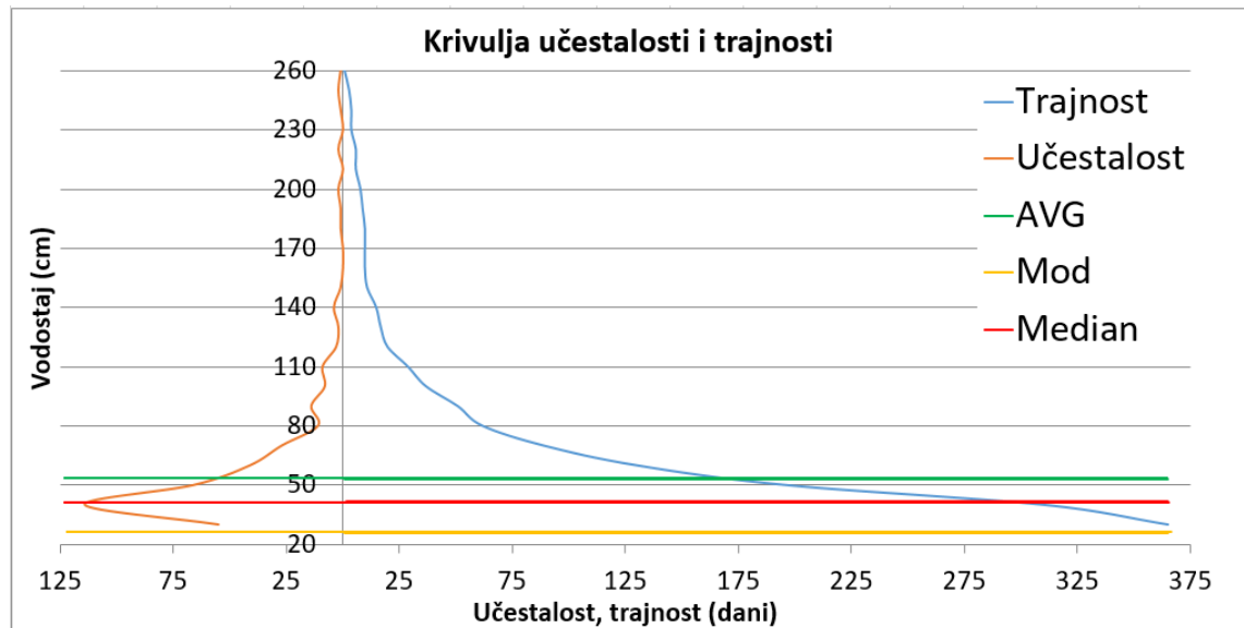
Slika 13. Grafički prikaz učestalosti i trajnosti vodomjerne stanice Ludbreg za 2019. godinu
