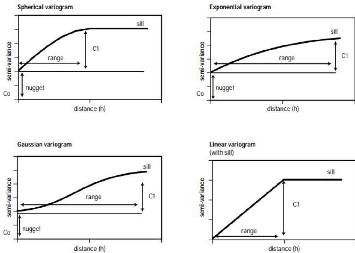
Slika 8. Teorijski variogramski modeli [20]
